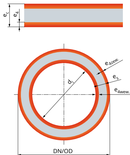
Przekrój rury strukturalnej z PVC-U typu A1
