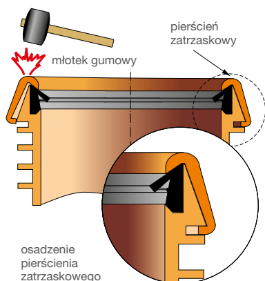
Uzbrajanie kielicha w uszczelkę
